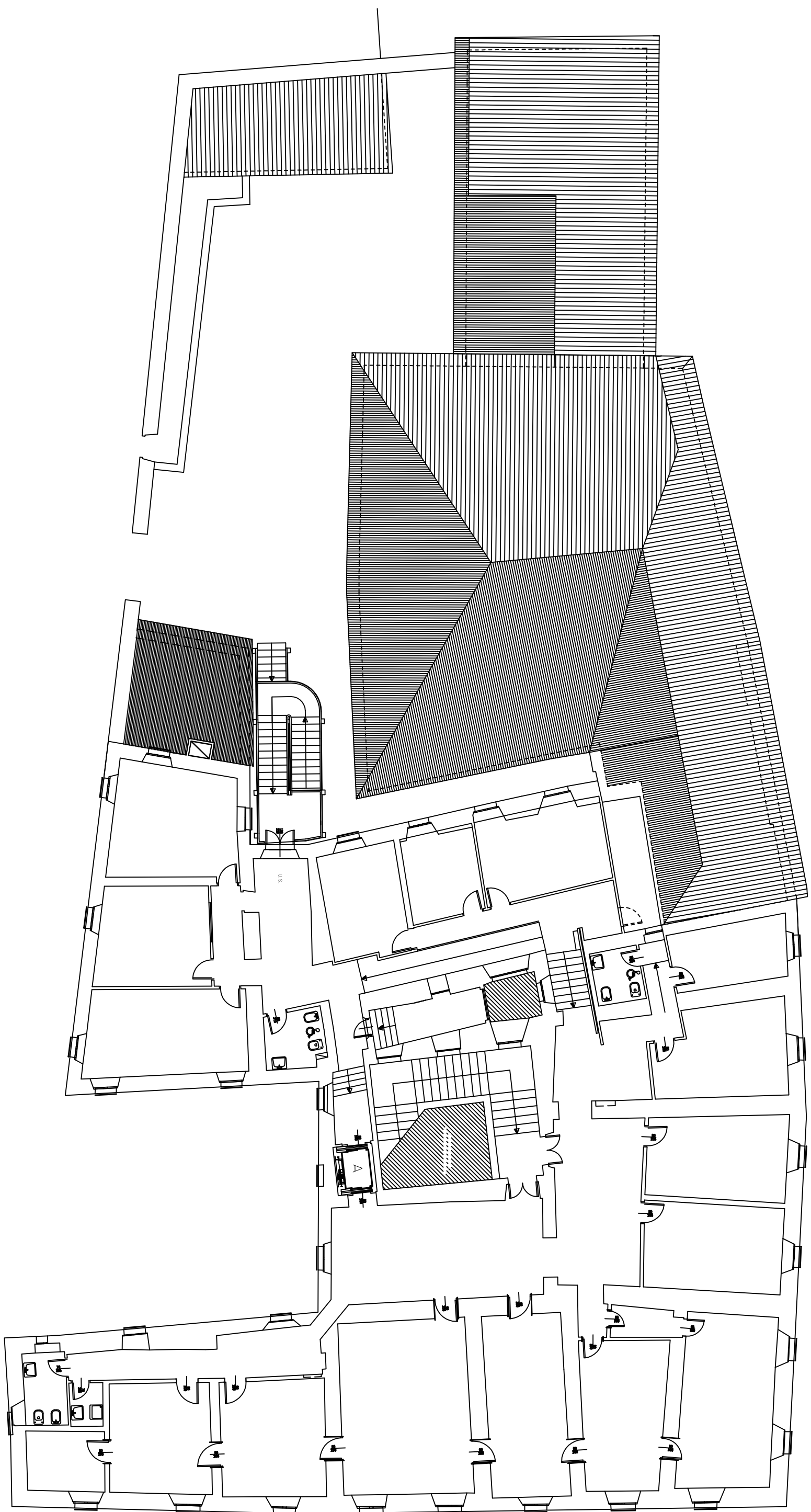
PALAZZO BATTIBOCCA LIVELLO 2 - PIANTA A QUOTA 960 - SECONDO PIANO
